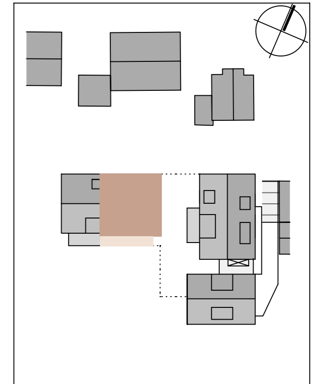
Grundriss Erdgeschoss M. 1:100
